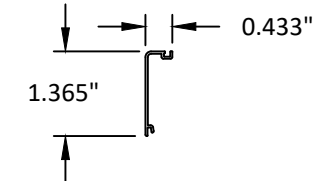
5 SASH END CAP 6063-T5
